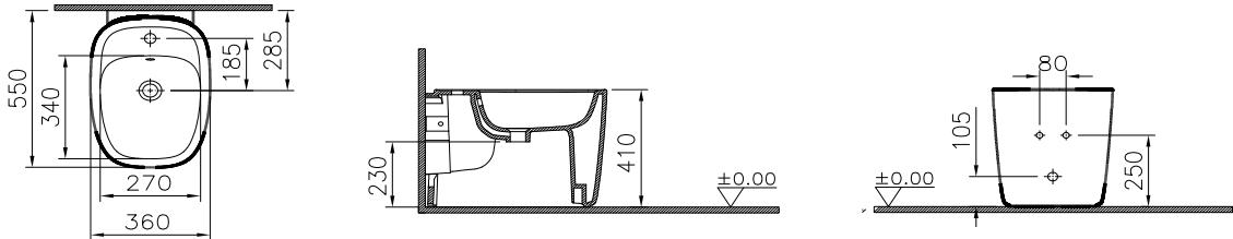
BIDET
