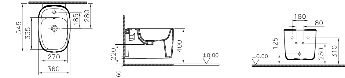
BIDET
